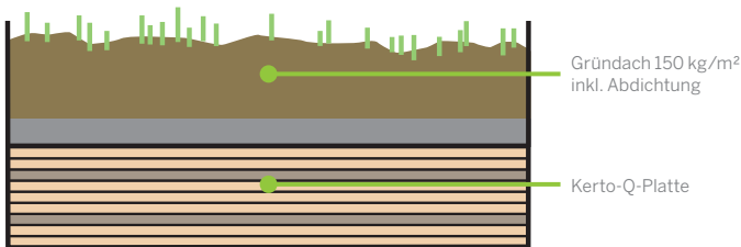
b) BEI GRÜNDACH g_{\text{Auf}} = 1,50 \text{ kN/m}^2
